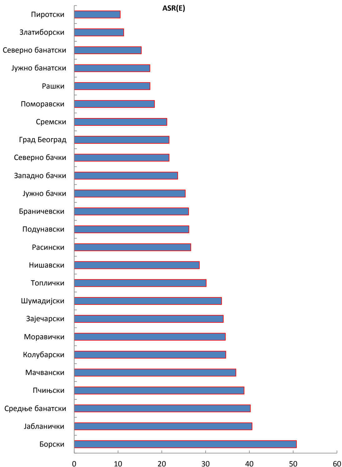
Табела 1. Стандардизоване стопе инциденције (*на популацију Европе) рака грлића материце, по округима у Републици Србији, 2013. година
